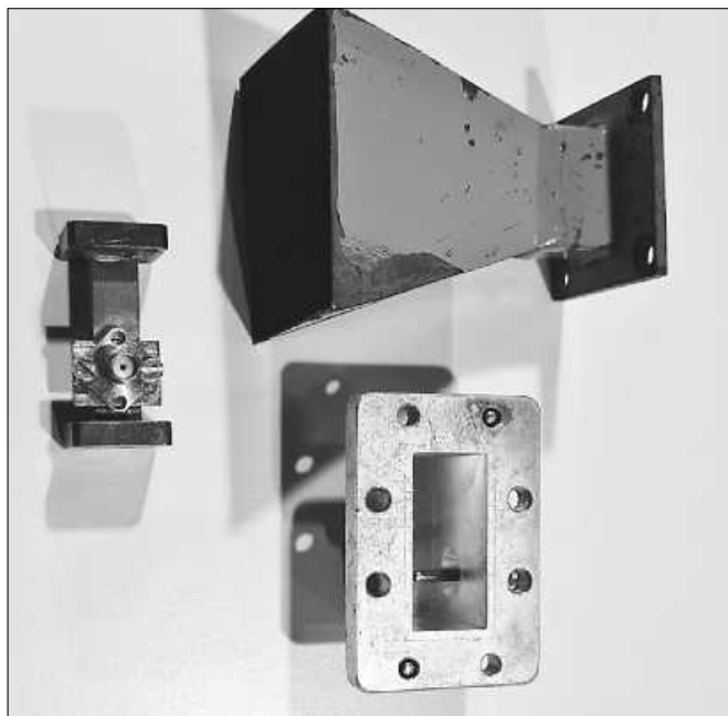
Hohlleiter und Antenne für sehr hohe Frequenzen im Gigahertz-Bereich.
