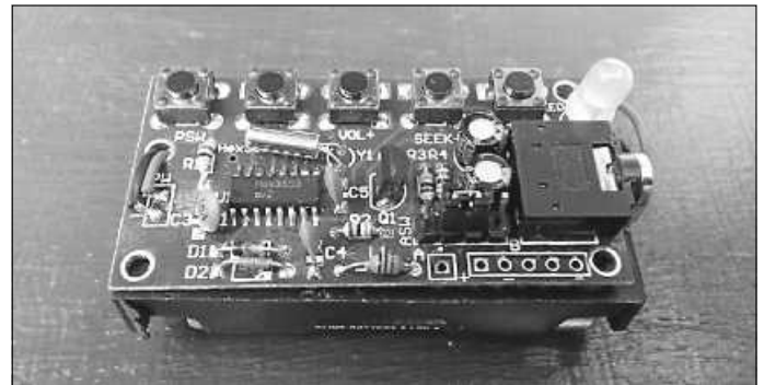
Mini FM-UKW-Radio
