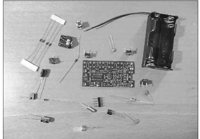
Elektronische Bauelemente aus denen ein UKW-Radio gebaut werden kann. Foto: JH
